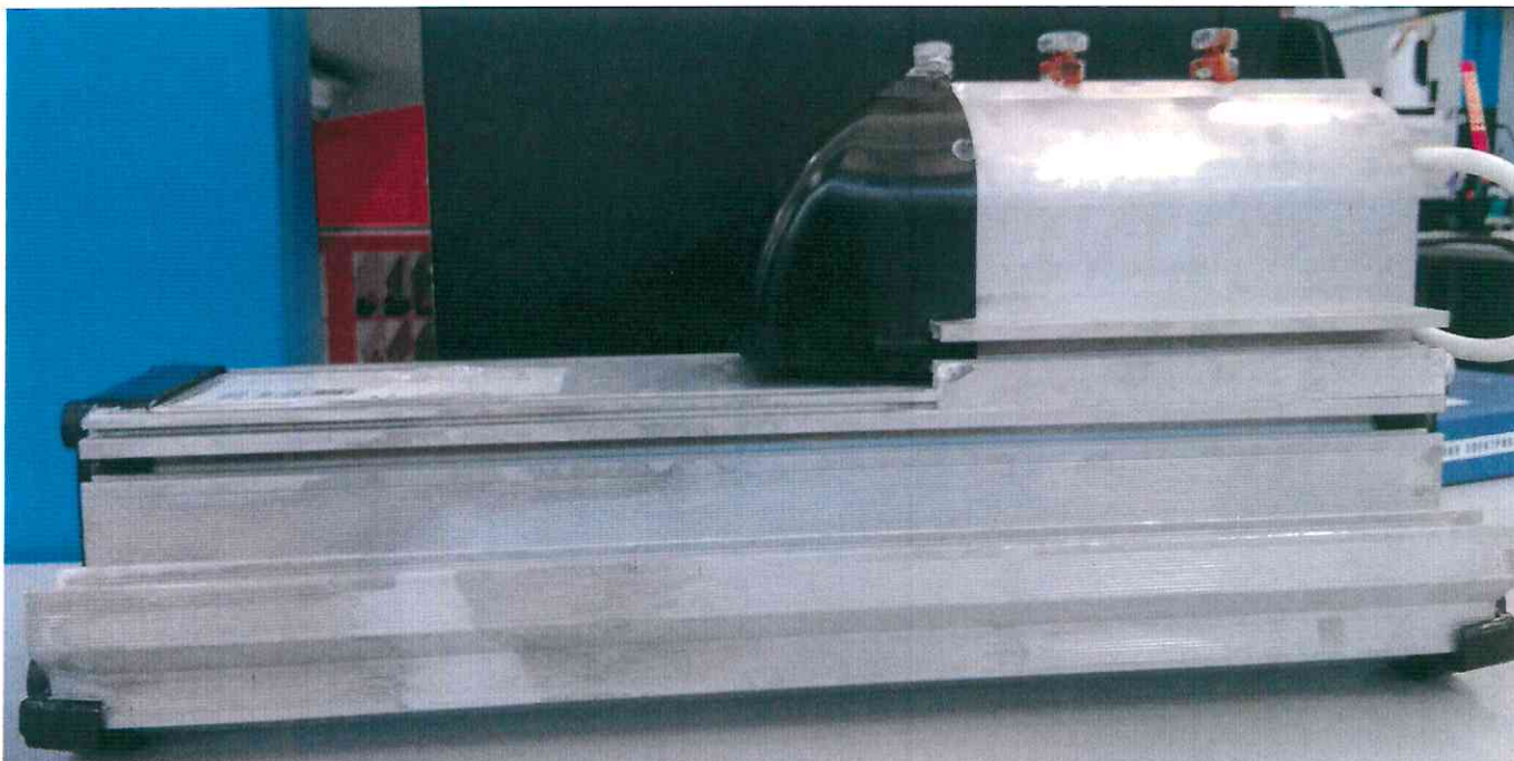
Рис.2. Фотография образца после испытаний
